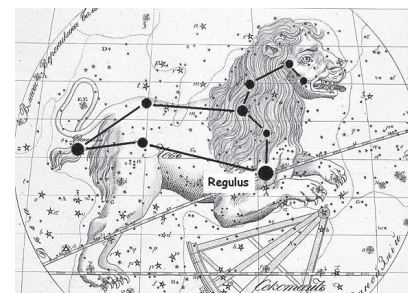
Das Sternbild Löwe Zeichnung von der Webseite: www.josef-bres-ser-sternwarte.de
